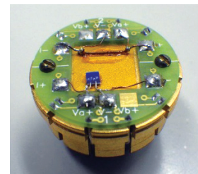
電気伝導測定用のホルダー
