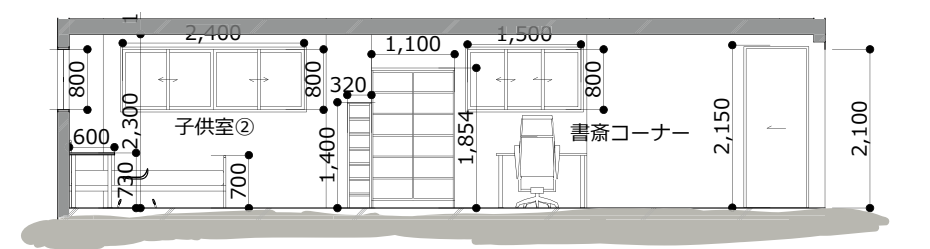
展開図 S=1/100
