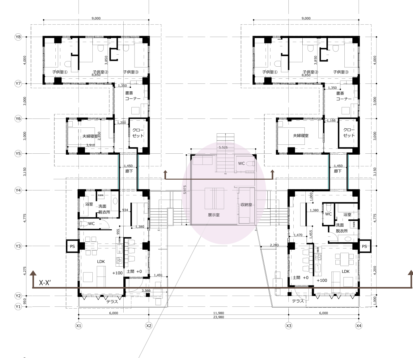
3階平面図 S=1/200
