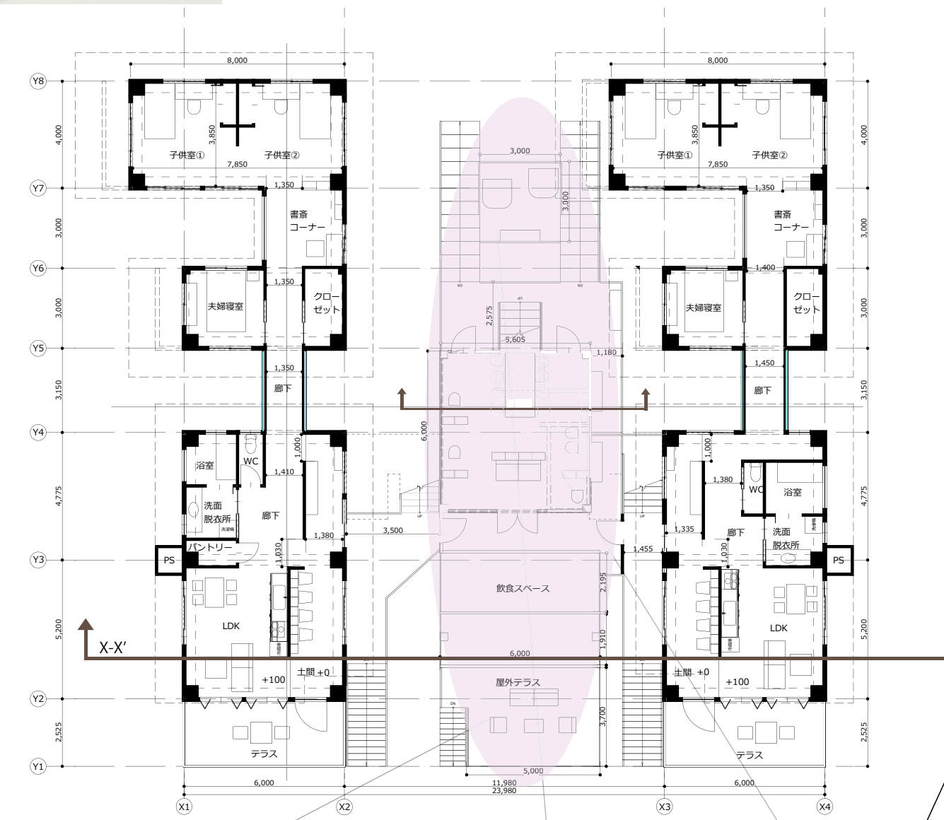
2階平面図 S=1/200
