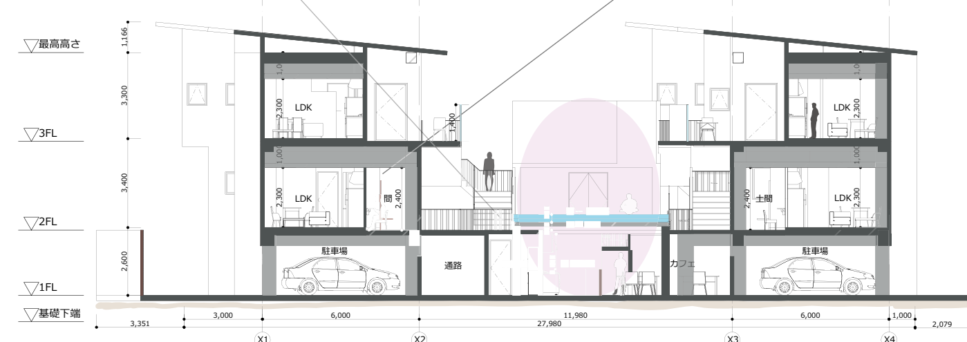
X-X' 断面図 S=1/200
