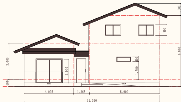
西側立面図 S 1:100
