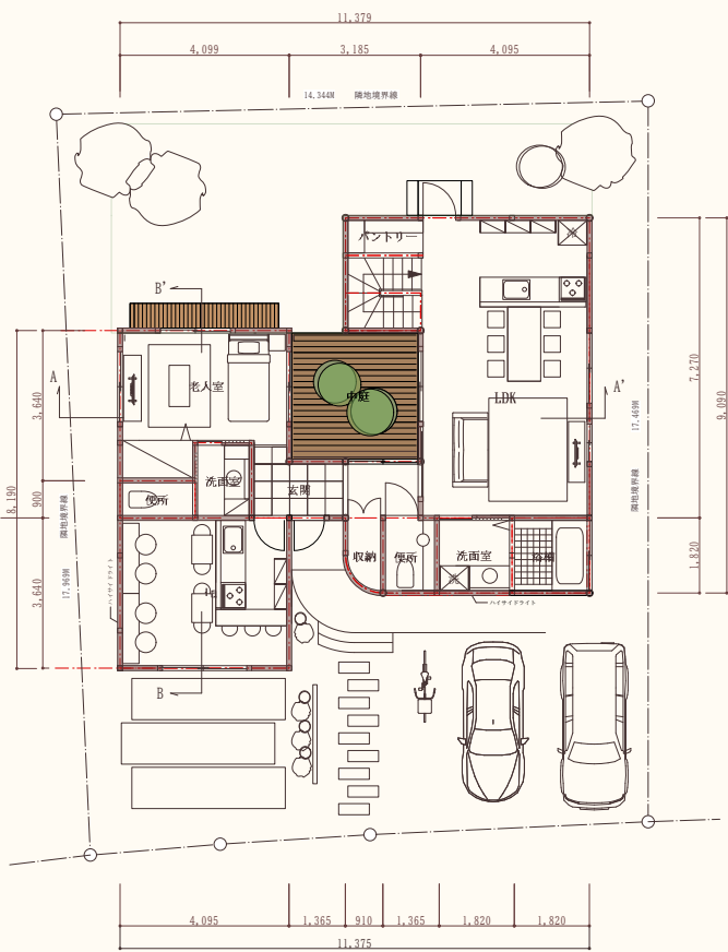
配置図兼一階平面図 S 1:100
